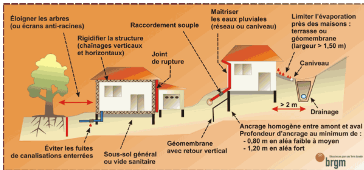
Exemples de dispositions préventives pour construire sur un sol argileux sujet au phénomène de retrait-gonflement
